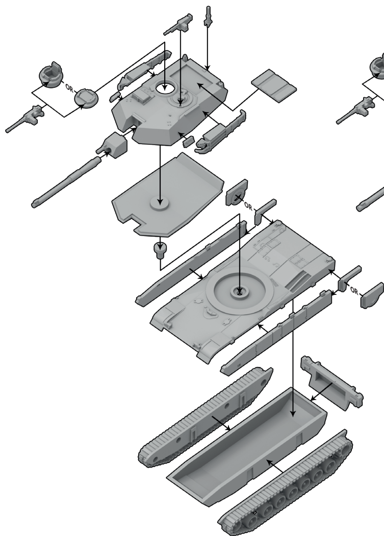
M1 ABRAMS
